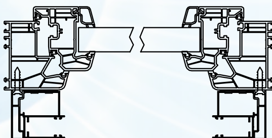
Profilo a "C" per predisposizione incasso 46 mm CON guida zanzariera Perfecta
