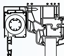
Profilo a "C" per predisposizione per incasso 46 mm CON cassonetto zanzariera Perfecta
