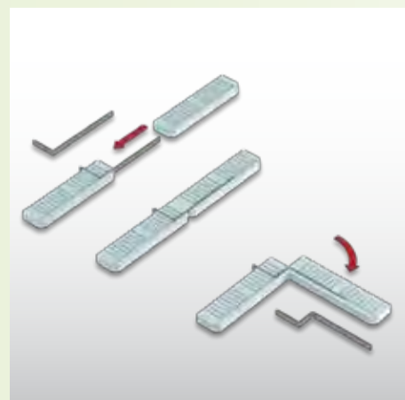
Le staffe a "zeta" modellabili. Con le apposite dime si può fare in cantiere.
