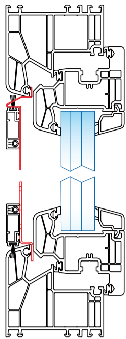
Clipfix, schema di installazione.
