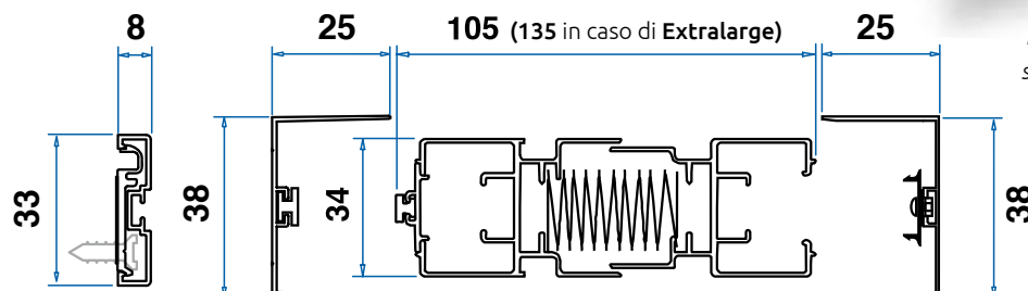
Profilo di riscontro ridotto (opzionale)
