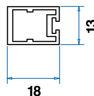
Profilo cornice a taglio 45° per attacco frontale
