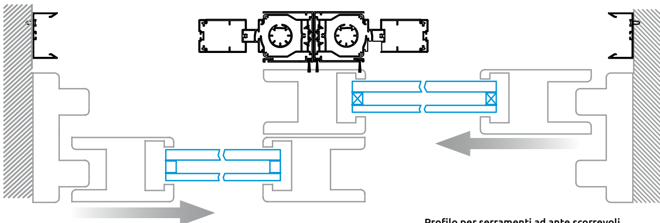
Profilo per serramenti ad ante scorrevoli, montaggio su anta doppia.
