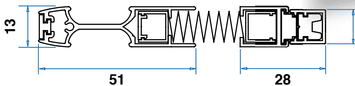
Barramaniglia + guida laterale (anta singola)
