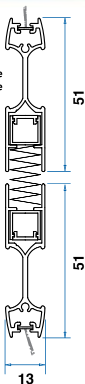
Barramaniglia e pacchetto rete
