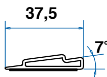
Guida a terra inclinata (opzionale)
