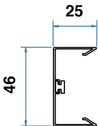
Guida superiore (Maxxy)
