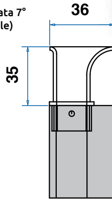
Deviatore per tapparella
