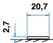
Guida a terra
