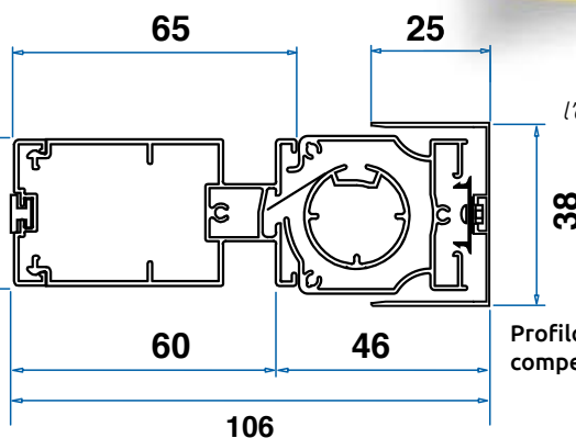
Pacchetto Rete con barramaniglia Maxxy
