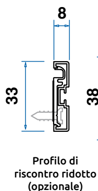
Barra di riscontro
