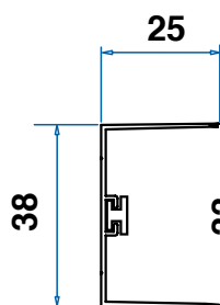
Barra di riscontro
