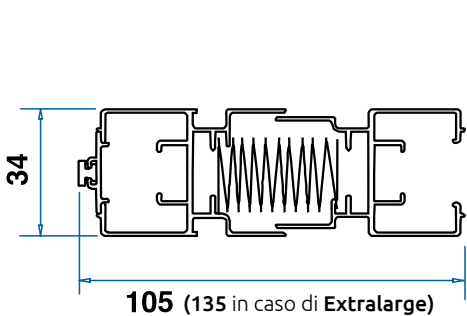
Barra di riscontro da incasso (Maxxy)
