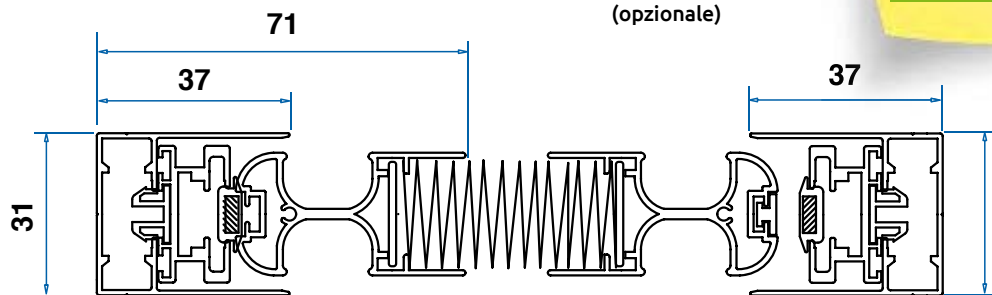
Profilo di riscontro
