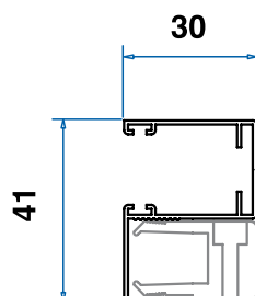
Guida 30x41
