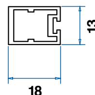
Profilo cornice a taglio 45° per attacco frontale
