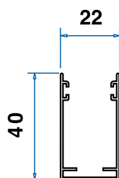
Guida 40x22
