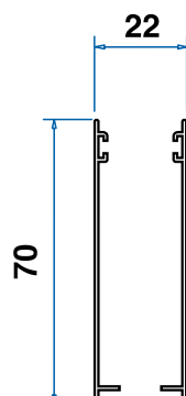
Guida 70x22
