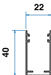
Guida 40x22
