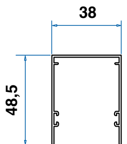
Guida superiore
