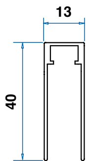
Guida superiore
