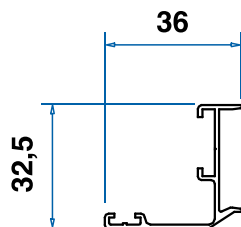
Profilo telaio
