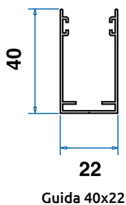
Guida 40x22
