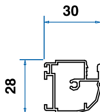
Profilo anta
