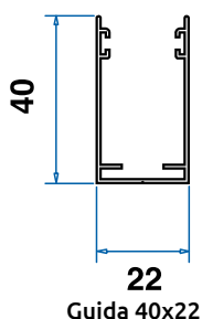
Guida 40x22
